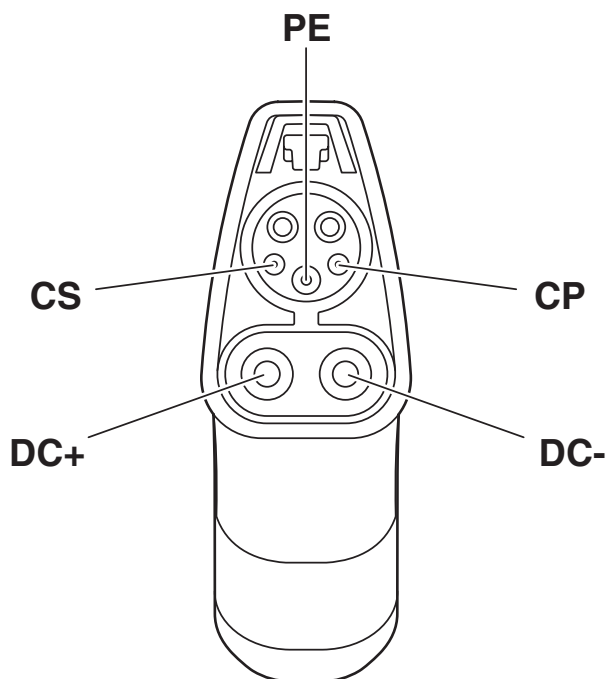
Schématický výkres
