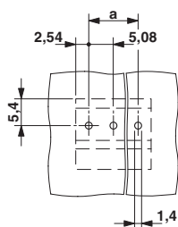
Vrtací schéma
