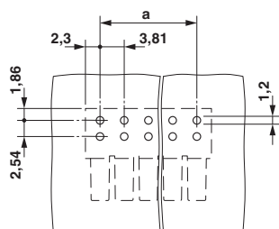
Vrtací schéma
