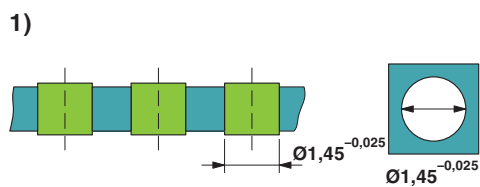
Vrtací schéma
