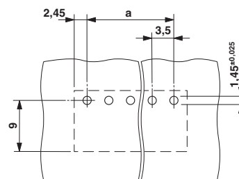
Vrtací schéma
