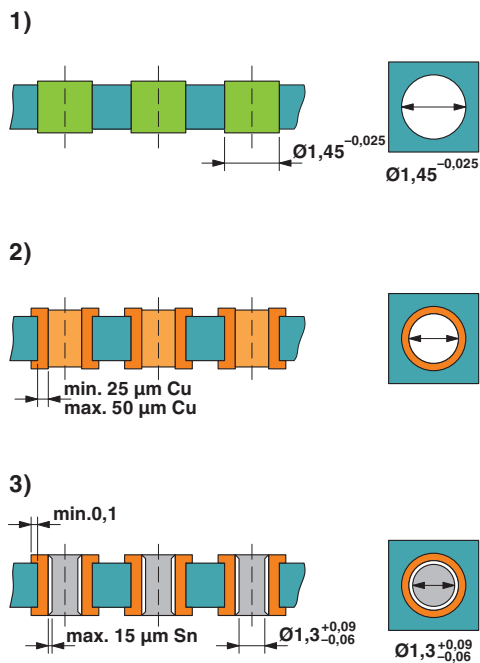
Vrtací schéma
