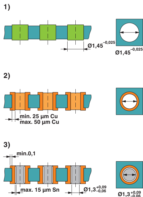
Vrtací schéma
