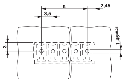
Vrtací schéma
