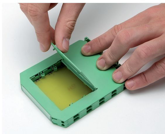
Sportello laterale aperto. Open side door.
