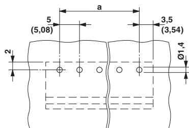
Vrtací schéma
