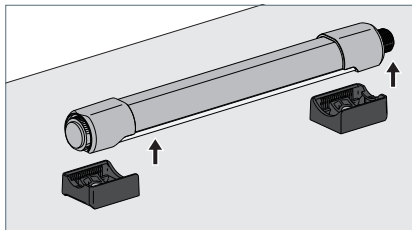
Fig. 10: Leuchte ausbauen.
